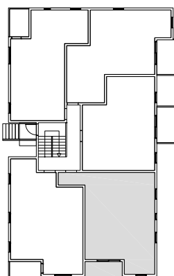
TLOCRT SUTERENA
